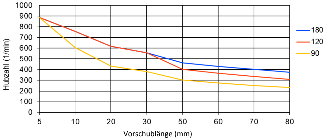
Hubzahldiagramm ohne Zwischenlüften mit Bandgewicht 0.1kg
