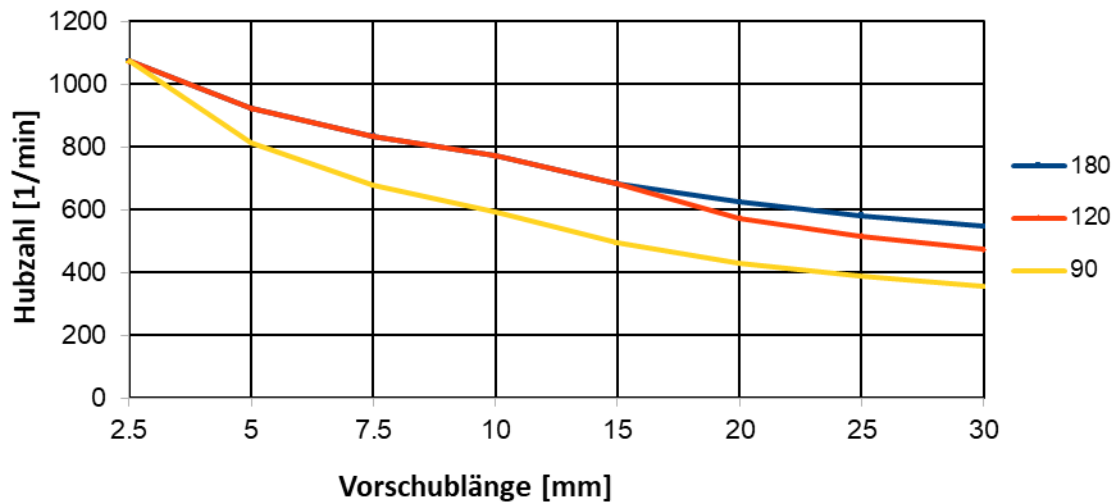
Hubzahldiagramm ohne Zwischenlüften mit Bandgewicht 0.1kg
