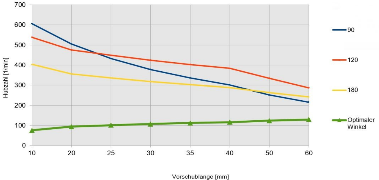
Hubzahldiagramm ohne Zwischenlüften mit Bandgewicht 0.5kg
